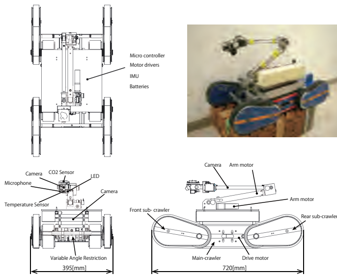
Fig. 28. CAD Drawings
