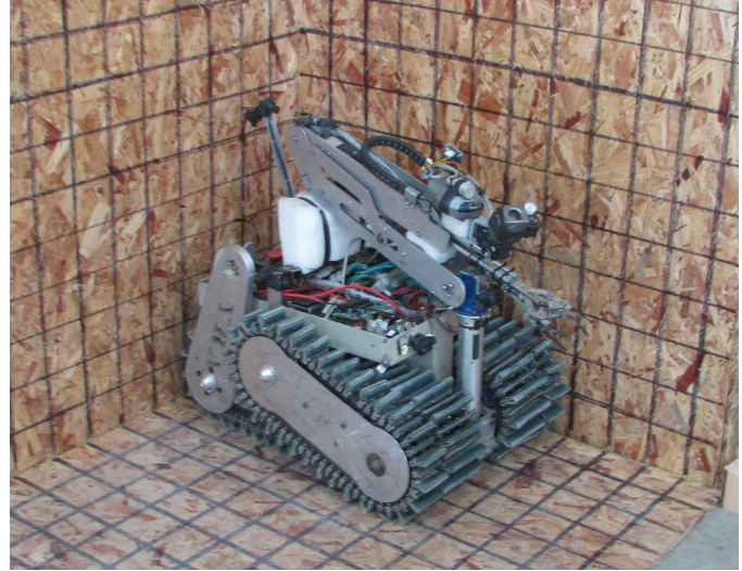
Fig. 1. YRA Tele Operationl Rescue Robot
